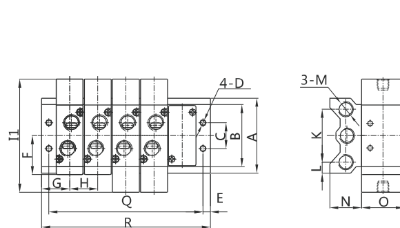
配4A系列气控阀
