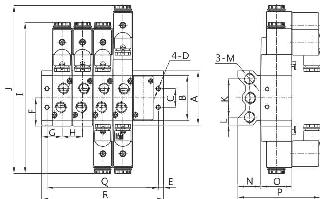
配4V系列电磁阀
